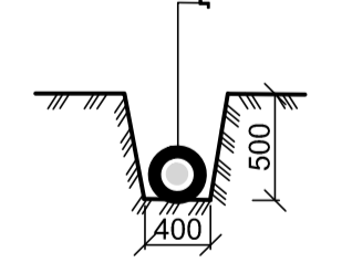
Сечение поливочного водопровода
